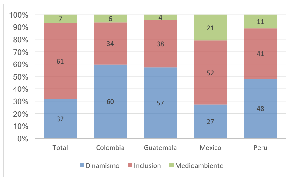
Figura 10: Descomposición Shorrocks-Shapley
