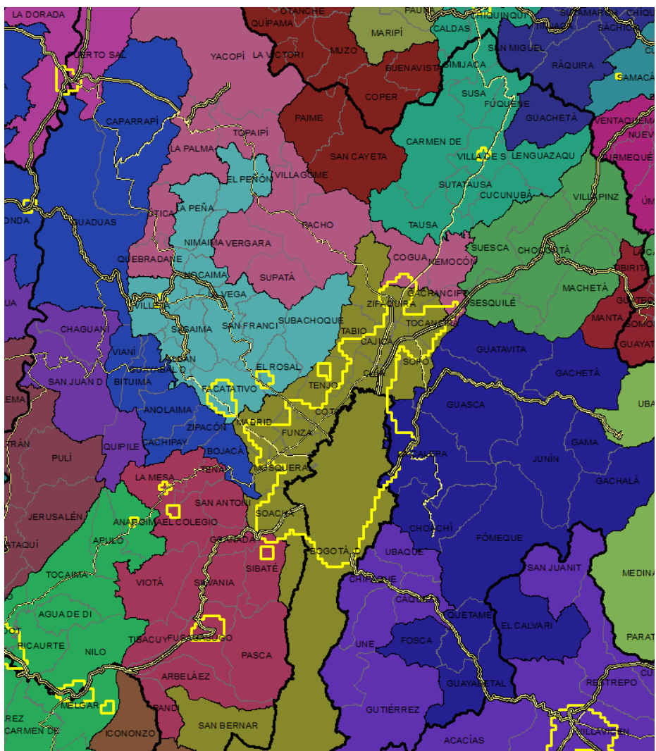
Figura 20. Subregionalización inicial aglomeración de Bogotá
